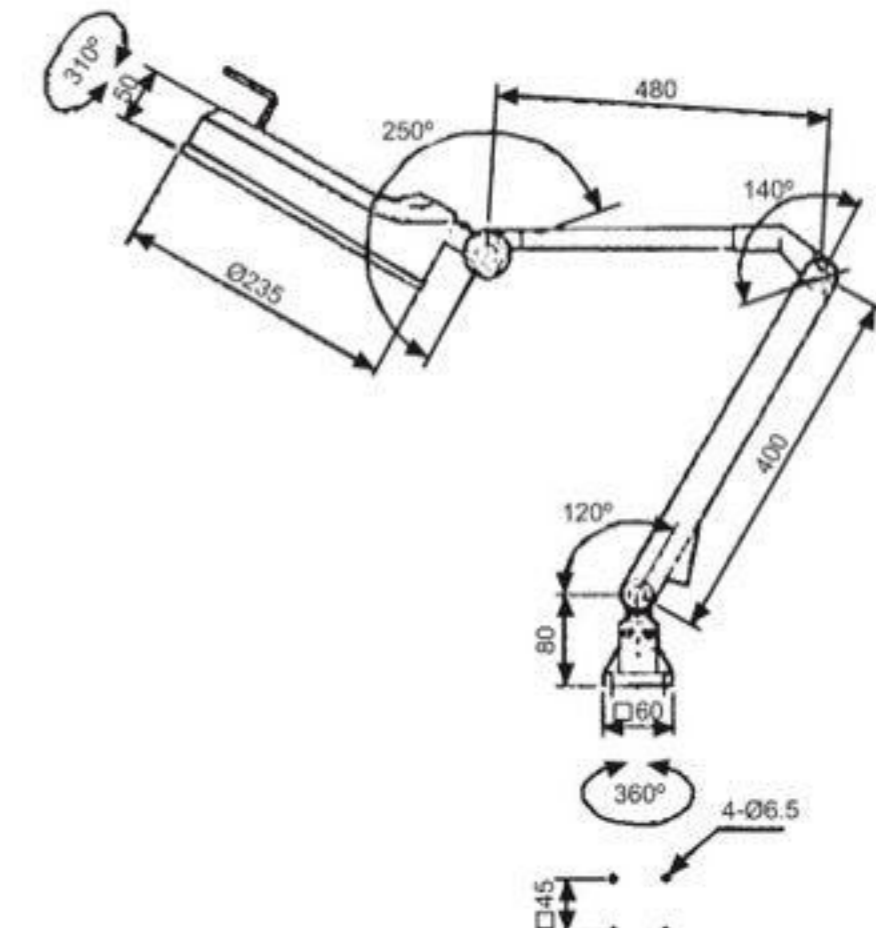
VHL-30LEB LONG ARM
