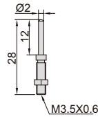
M3.5X0.6
