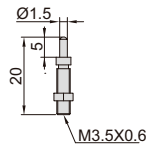
M3.5X0.6
