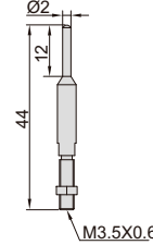
M3.5X0.6
