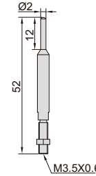
M3.5X0.6
