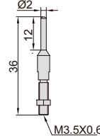
M3.5X0.6
