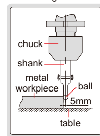
X-Y edge finder
