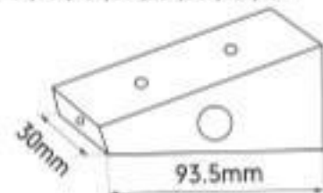
BASE PLATE 5°, 10°, 15°, 20°, 25°, 30°, 40°, 45°
