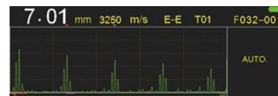
A-Scan
