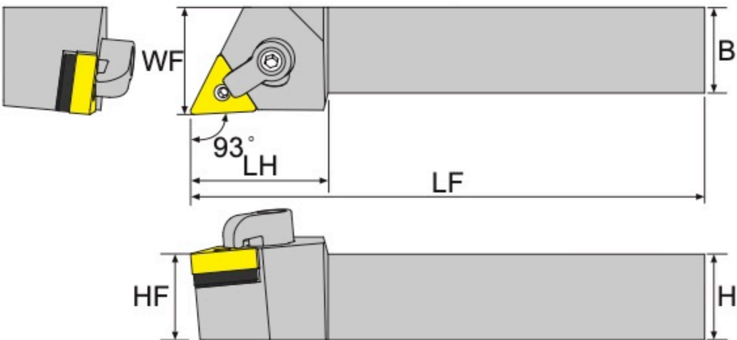
Dimension(mm)
