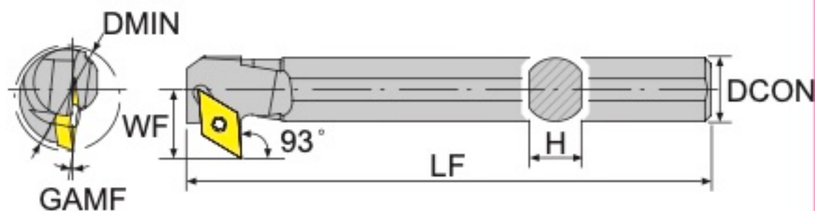
內徑加工車刀 Boring Bar
