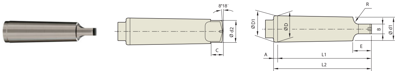
DIN 228 (MORSE TAPER) TANG TYPE (MTA)
