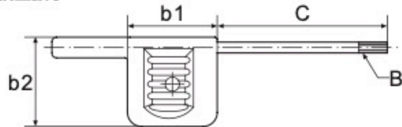
旗型扳手
