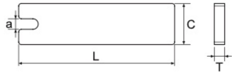
鑰型扳手
