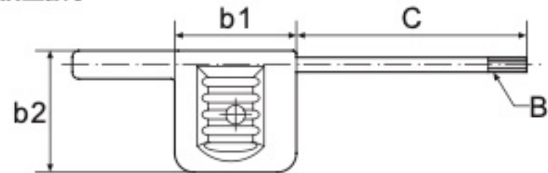
旗型扳手
