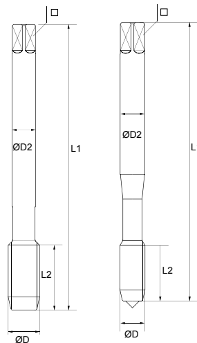
Shank: DIN 376
