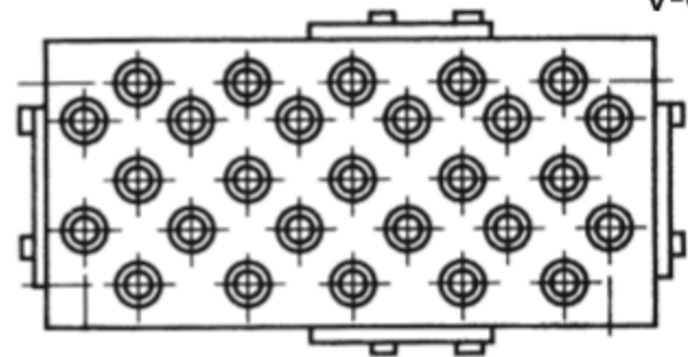
V-47S, V-66S M6 X 1.0
