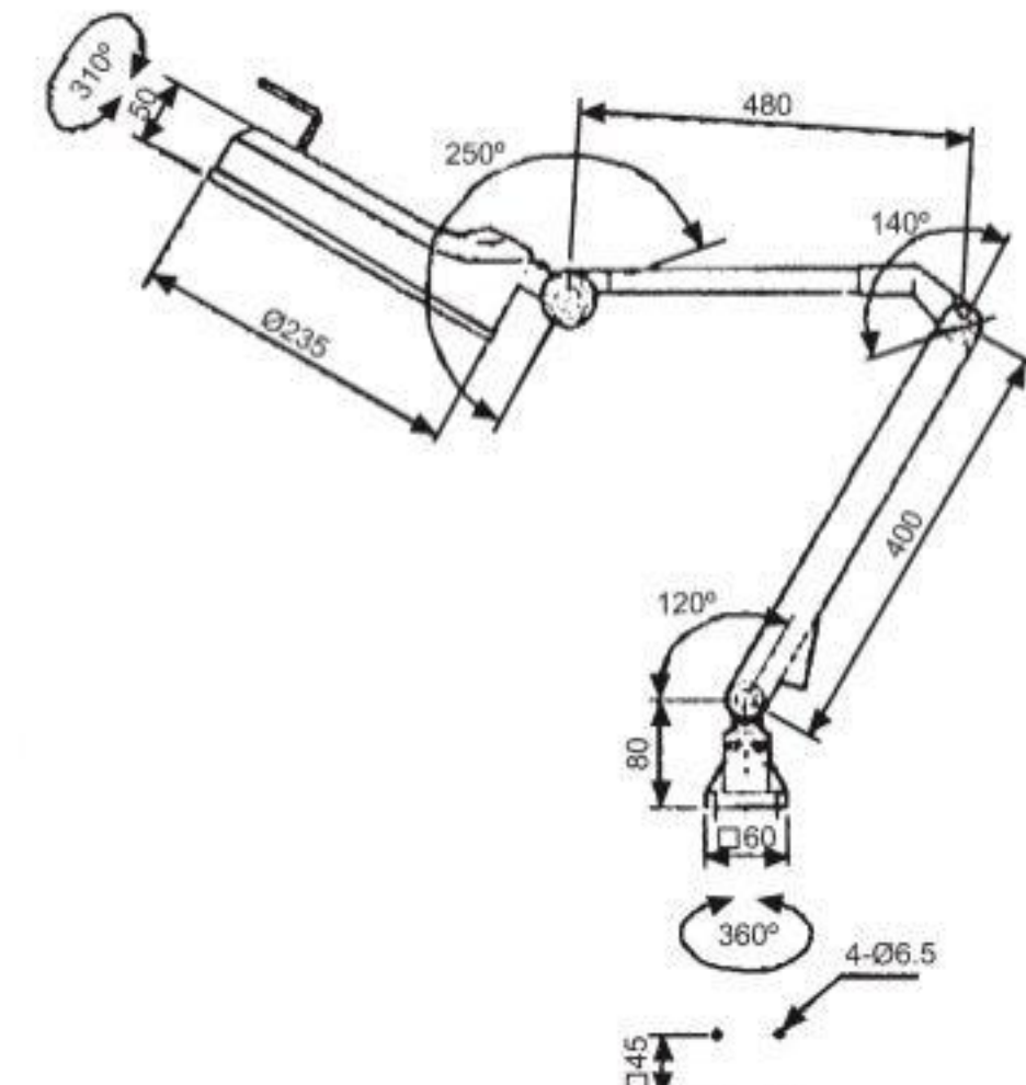
VHL-30LEB LONG ARM
