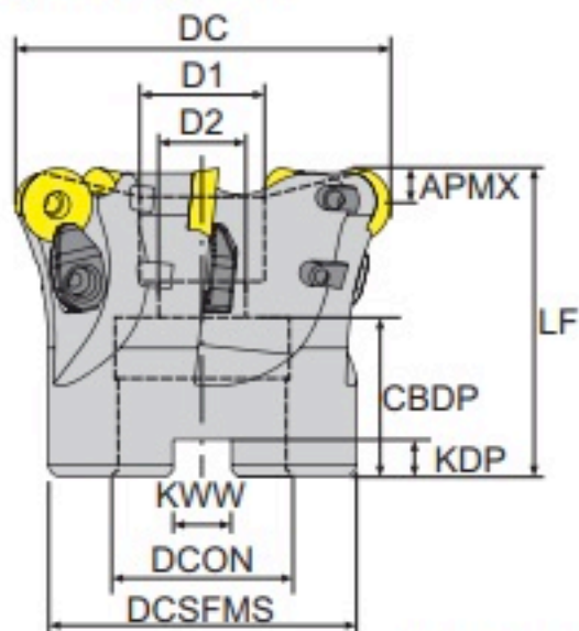
寸法 Dimension(mm)
